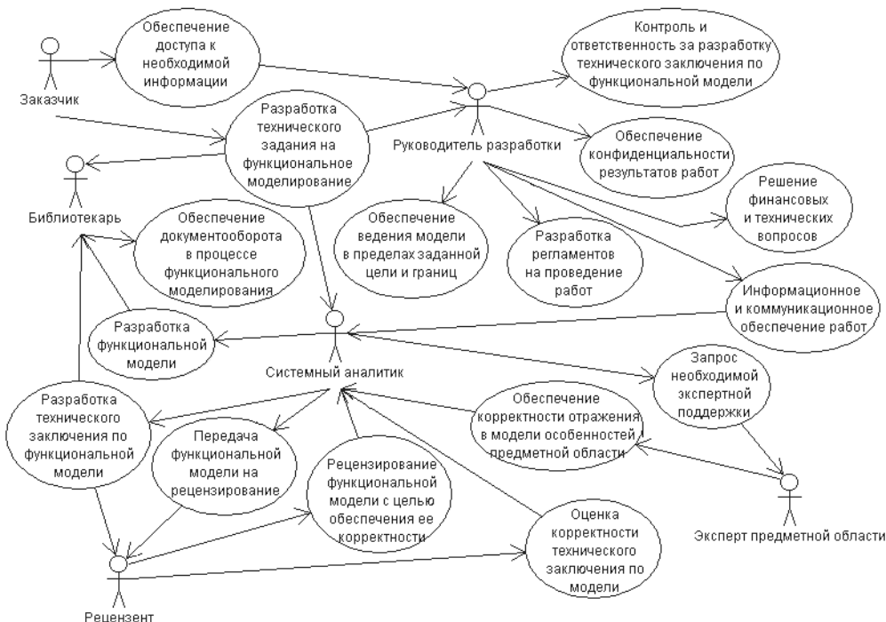
Рис. 2. Схема организации работ по функциональному моделированию информационных систем в графической нотации UML
