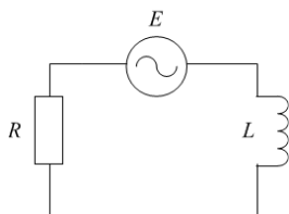
Рис. 2. Электрическая цепь
