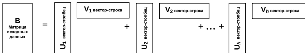
Рис. 1. Схема факторизации в диадном анализе
